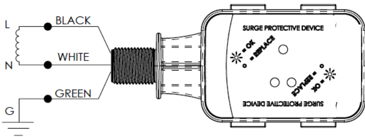
PQLA 120/240
